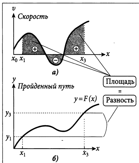
Рис. 2. Графики скорости и пути.
