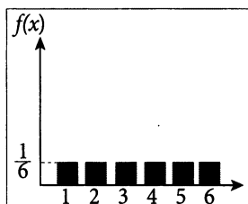
Рис. 4. Функция плотности вероятности.
