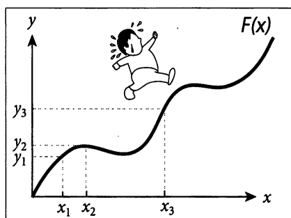
Рис. 1. График зависимости пройденного Футоши пути от времени. Он проходит точки y_1, y_2, y_3... в моменты времени x_1, x_2, x_3...
