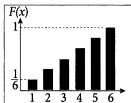
Рис. 5. Функция распределения вероятности.
